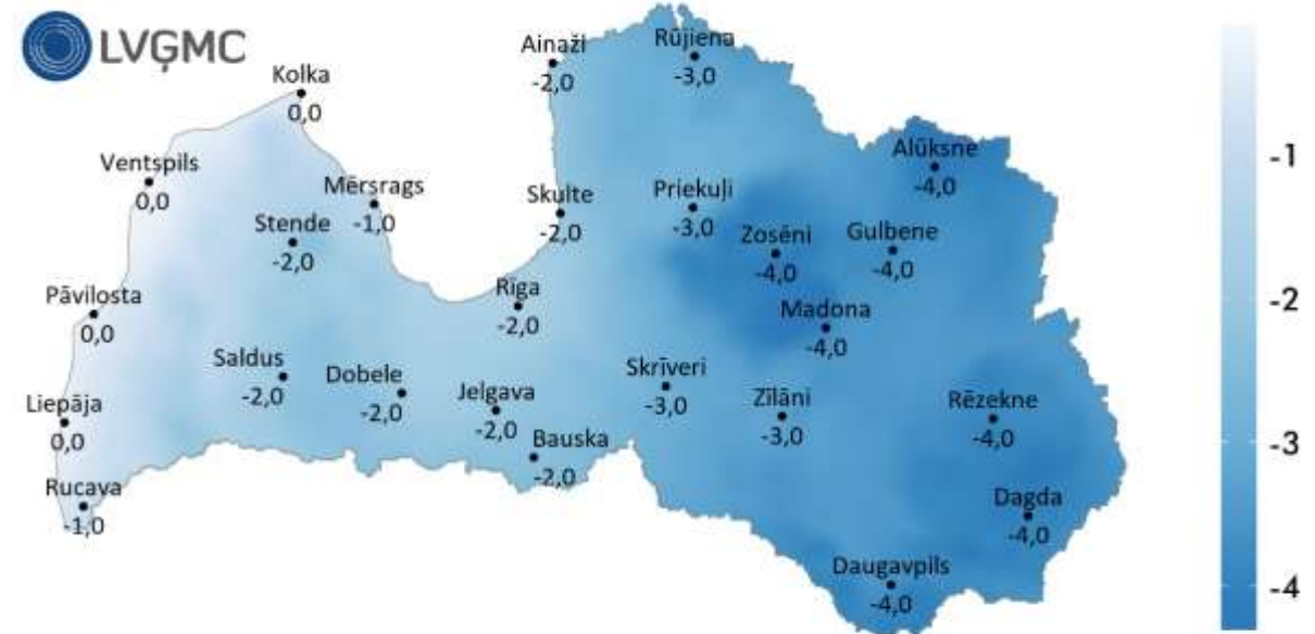
Ziemas klimatiskā norma Latvijā, 1991.-2020. gads, °C
